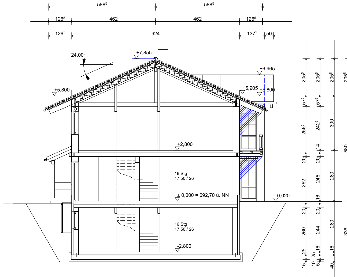
Schnitt 3 - 3 Haus 4
