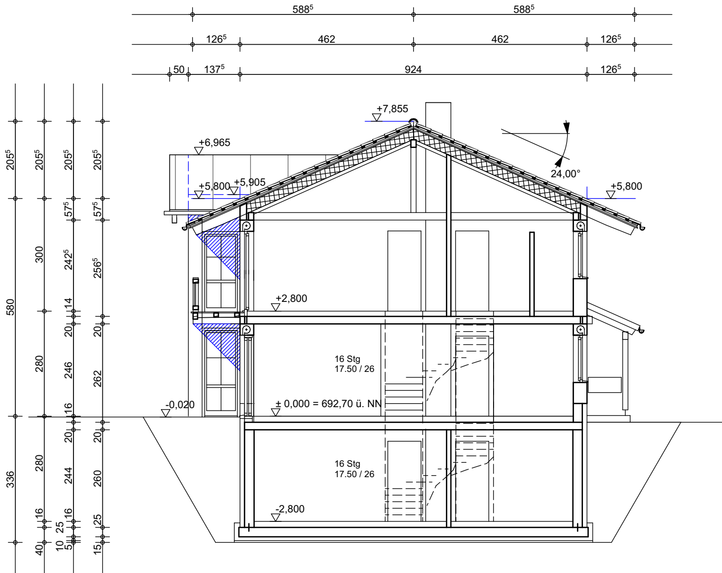
Schnitt 2 - 2 Haus 3
