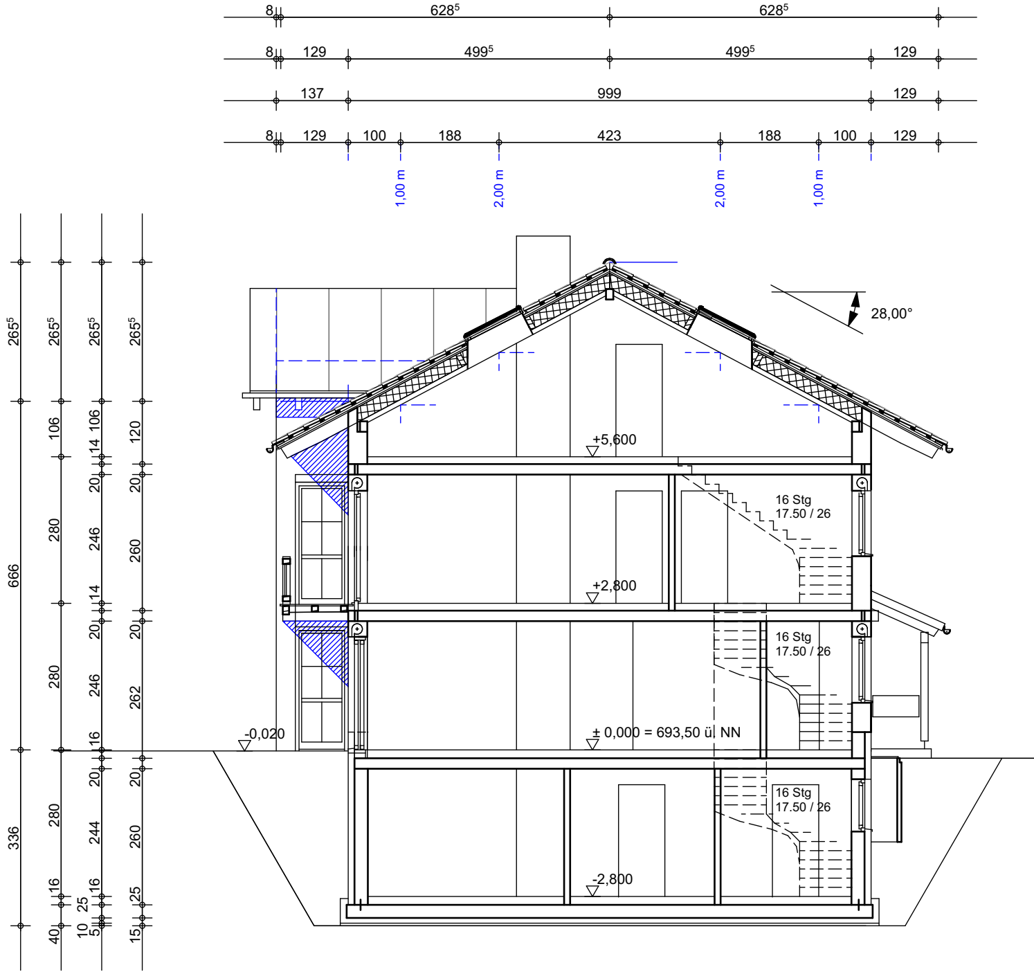
Schnitt 1 - 1 Haus 2 ( Haus 1 analog )
